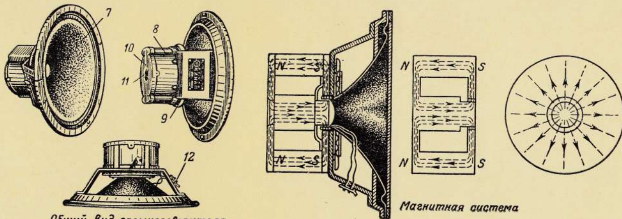
Общий вид громкоговорителя
