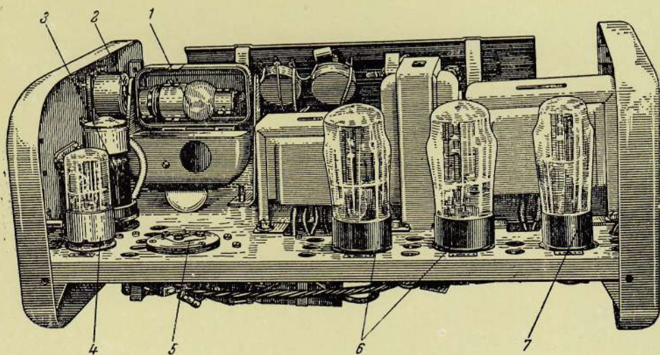
Вид со стороны подъемного винта и со стороны ламп (со снятой крышкой)
