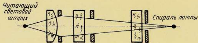
Схема хода лучей в двух главных сечениях цилиндрической оптики
