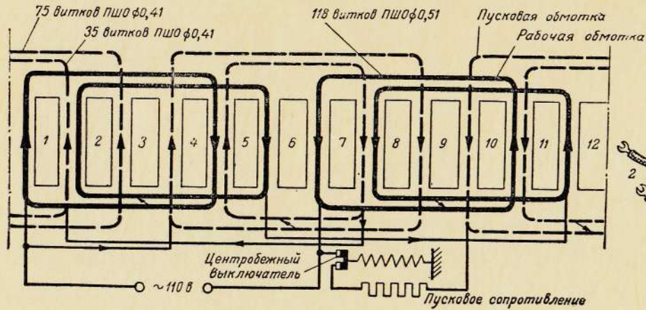
Электрическая схема электродвигателя
