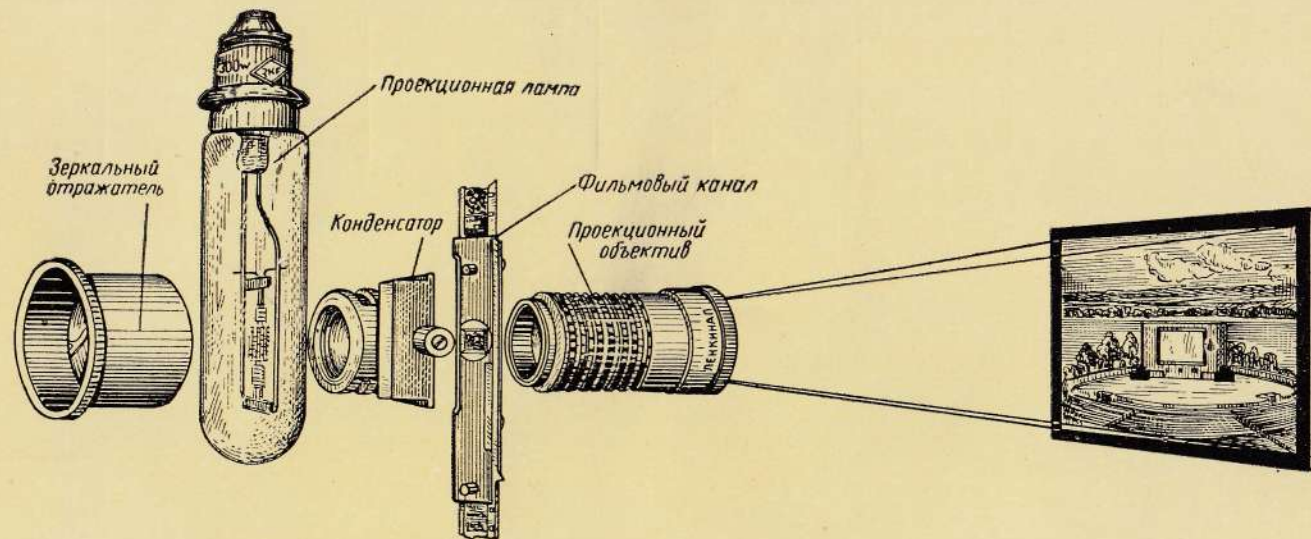
Схема оптики
