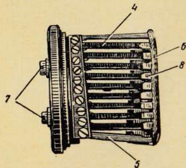
Внутренний вид (снизу)
