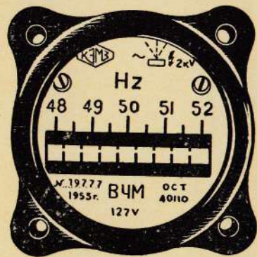
Общий вид
