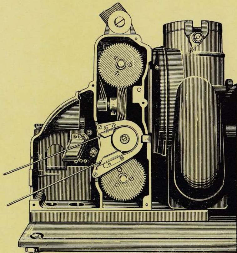
Вид со стороны механизма передач
