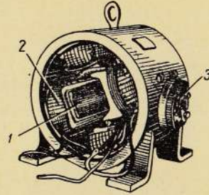
Станина генератора
