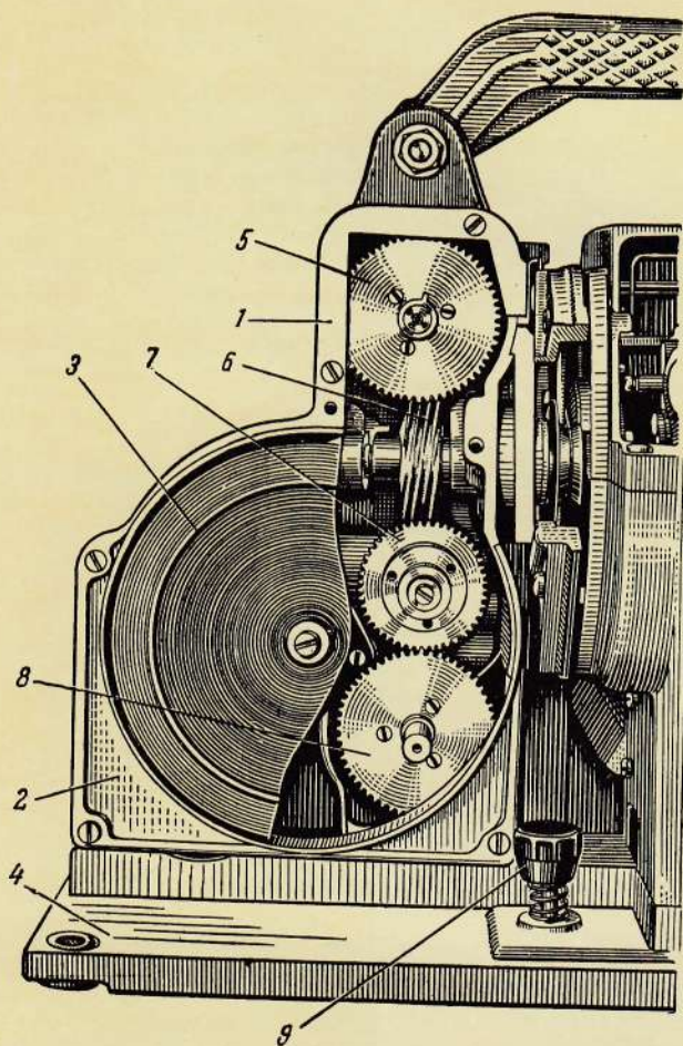
Вид со стороны передаточного механизма
