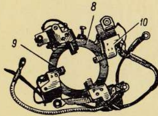
Траверса
