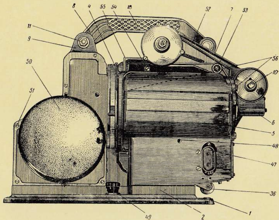
Вид с нерабочей стороны
