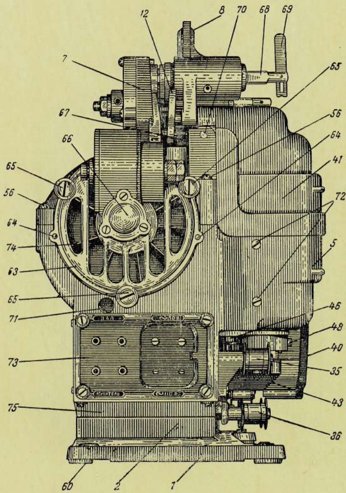
Вид со стороны клеммного плато
