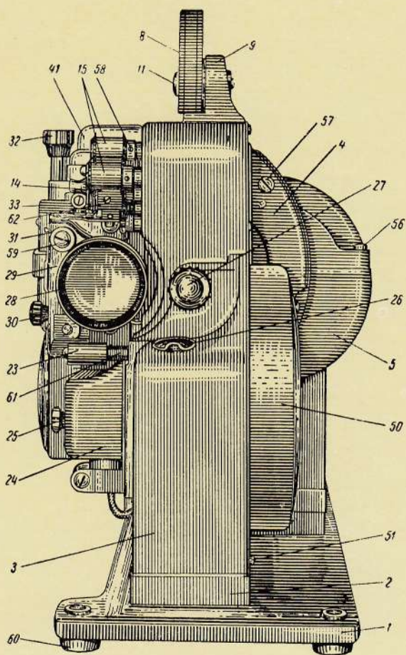
Вид со стороны объектива
