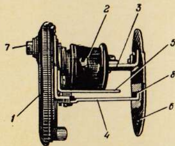
Внутренний вид (сверху)
