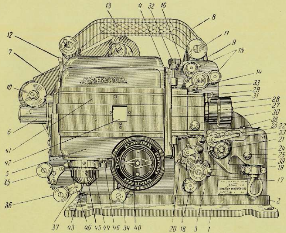
Вид с рабочей стороны
