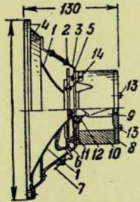
Конструкция
