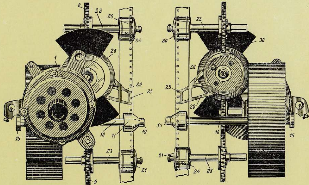
Вид со стороны электродвигателя
