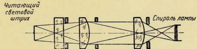
Схема хода лучей в двух главных сечениях цилиндрической оптики
