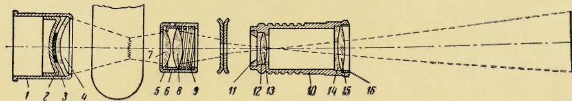
Схема оптики
