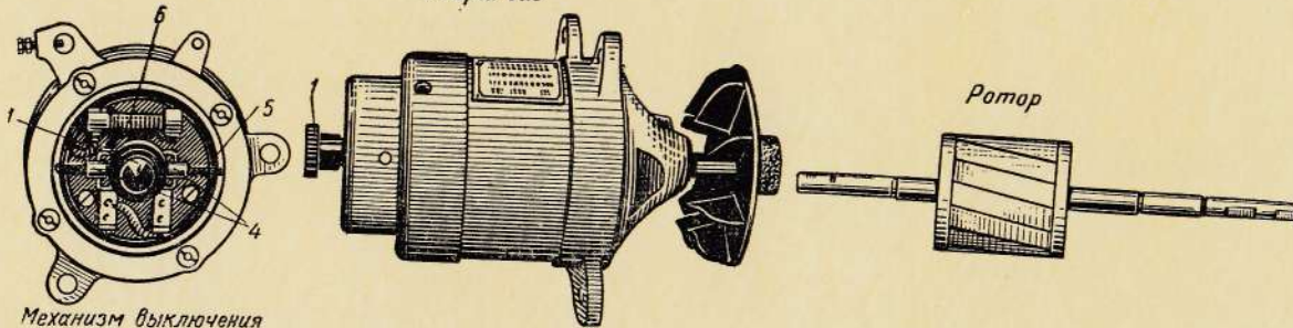
Механизм выключения пусковой обмотки
