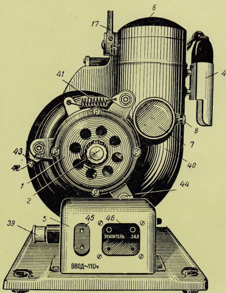
Вид со стороны электродвигателя
