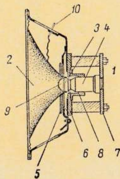
Разрез
