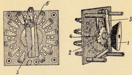
Конструкция переключателя
