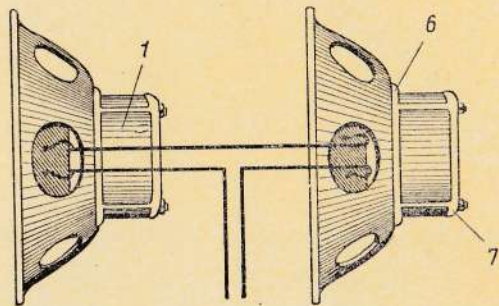
Соединение громкоговорителя
