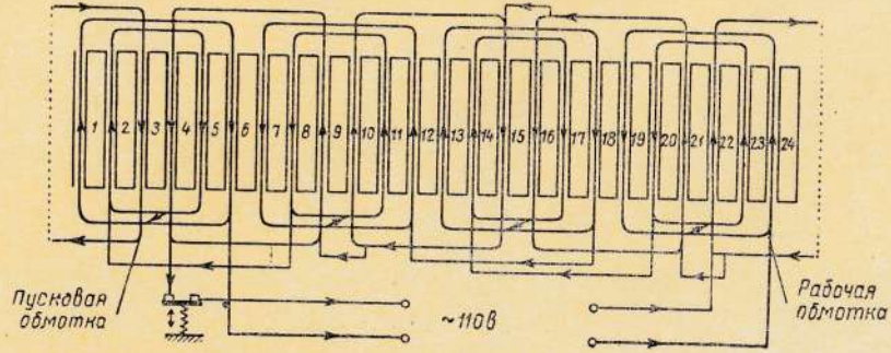
Электрическая схема обмоток
