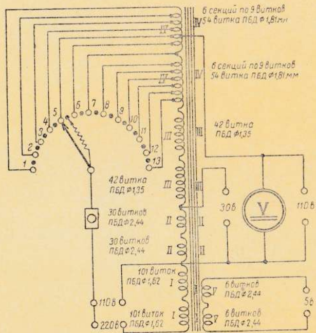
Принципиальная электрическая схема
