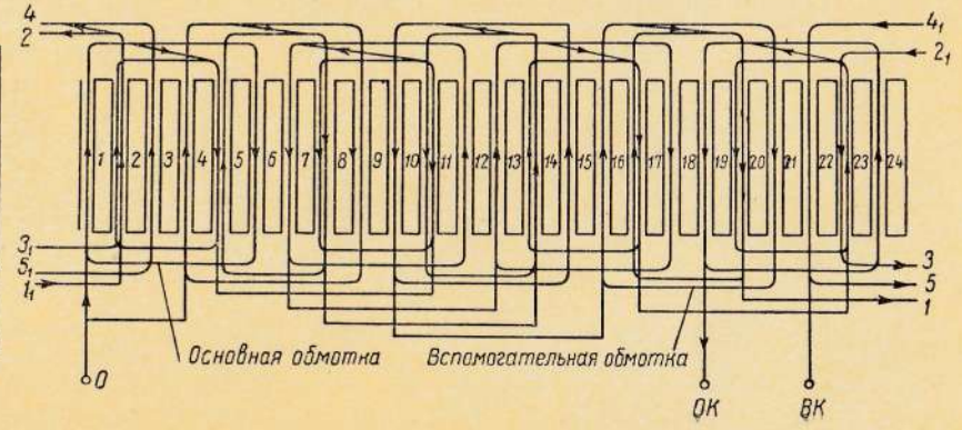
электрическая схема обмоток
