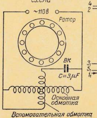
Принципиальная электрическая схема
