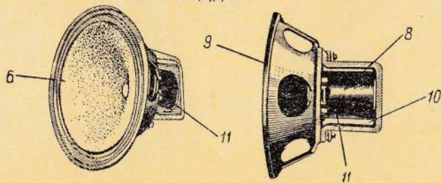
Головка ГДД-157
