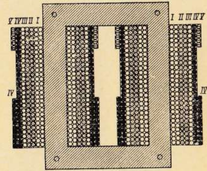
Расположение обмоток
