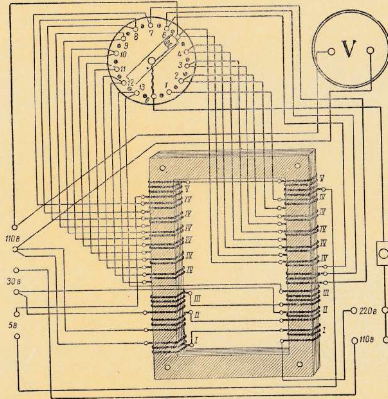
МОНТАЖНАЯ СХЕМА
