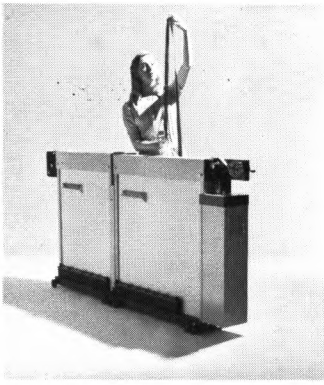
КОМБИЛАБОР: АВТОМАТИЧЕСКАЯ ПРОЯВОЧНАЯ МАШИНА ДЛЯ 16-ММ И 35-ММ ЧЁРНО-БЕЛЫХ ПОЗИТИВНЫХ И НЕГАТИВНЫХ ИЛИ ОБРАТИМЫХ КИНОПЛЁНОК.
