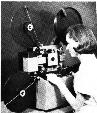
КОПИЛИКС: КОПИРОВАЛЬНАЯ МАШИНА ДЛЯ КОПИРОВАНИЯ 35-ММ ПЛЁНОК НА 16-ММ ПЛЁНКИ И 16-ММ ПЛЁНОК НА ТОТ ФОРМАТ.
