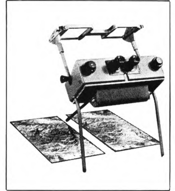
О Д С С: СИСТЕМА СТЕРЕО-СКАНИРОВАНИЯ ДЛЯ АНАЛИЗА СНИМКОВ, СДЕЛАННЫХ С ВОЗДУХА.
