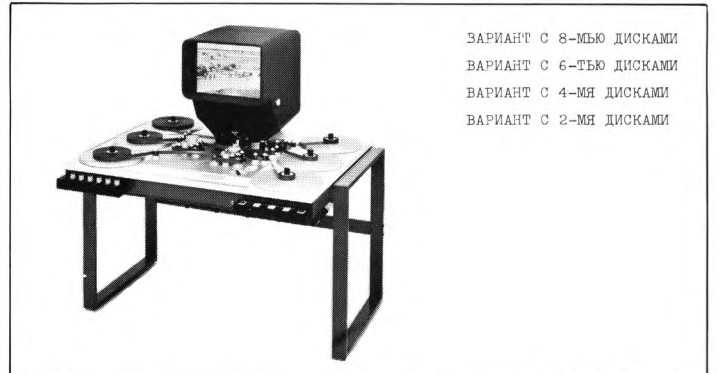
СИНЕМОНТА: ГОРИЗОНТАЛЬНЫЙ МОНТАЖНЫЙ СТОЛ ДЛЯ 16-ММ И 35-ММ КИНОПЛЁНОК.
