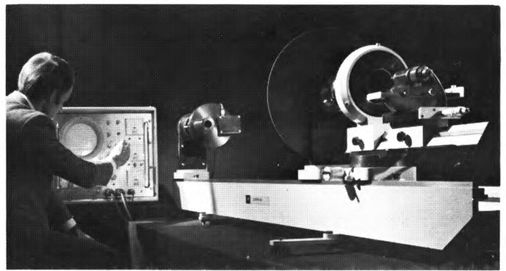
ОЛЕТА: УСТРОЙСТВО ДЛЯ ИЗМЕРЕНИЯ КОЭФФИЦИЕНТА ПЕРЕНОСА ДЛЯ ОПТИЧЕСКИХ И ЭЛЕКТРО-ОПТИЧЕСКИХ СИСТЕМ.
