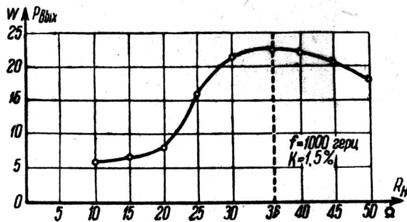
Рис. 9. Нагрузочная характеристика усилителя 1У-45
