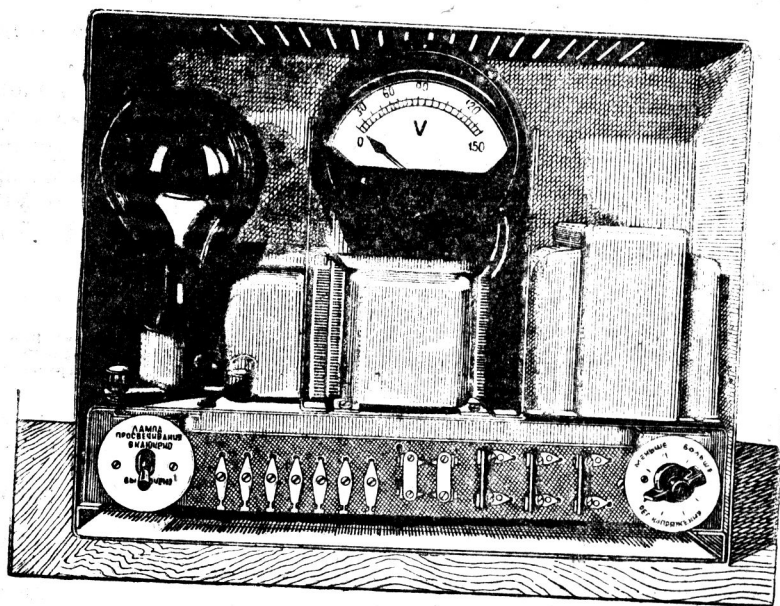
Рис. 18. Выпрямитель 1В-45 (вид со снятой крышкой)
