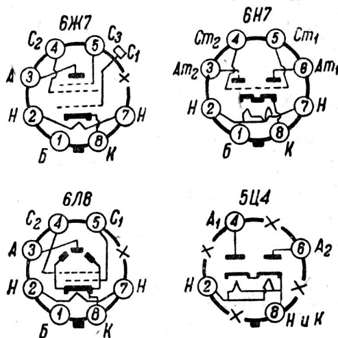
Рис. 3. Цоколевка ламп (вид снизу)
