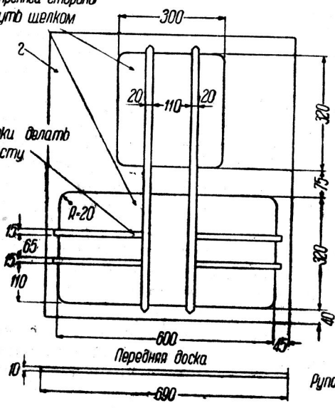
Рис. 21. Рупор РСД-2М
