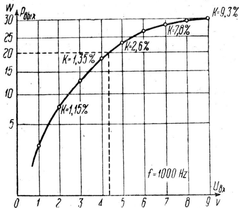
Рис. 6. Амплитудная характеристика усилителя 1У-45
