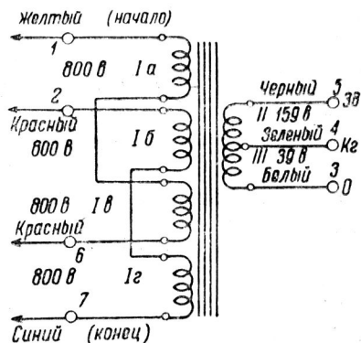
Рис. 5. Схема обмоток выходного трансформатора усилителя 1У-45
