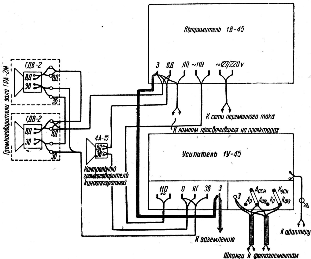
Рис. 28. Схема соединения аппаратуры одного комплекта УСУ-45
