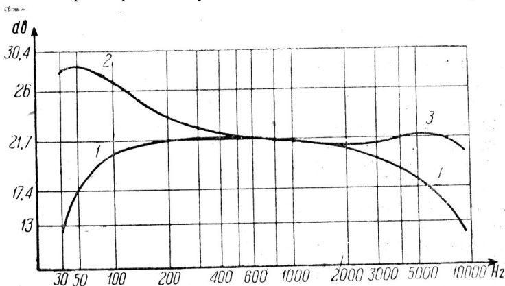
Рис. 8. Частотные характеристики усилителя 1У-45
