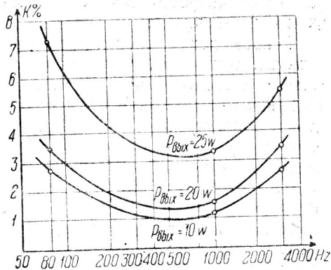
Рис. 7. Характеристики клирфактора усилителя 1У-45
