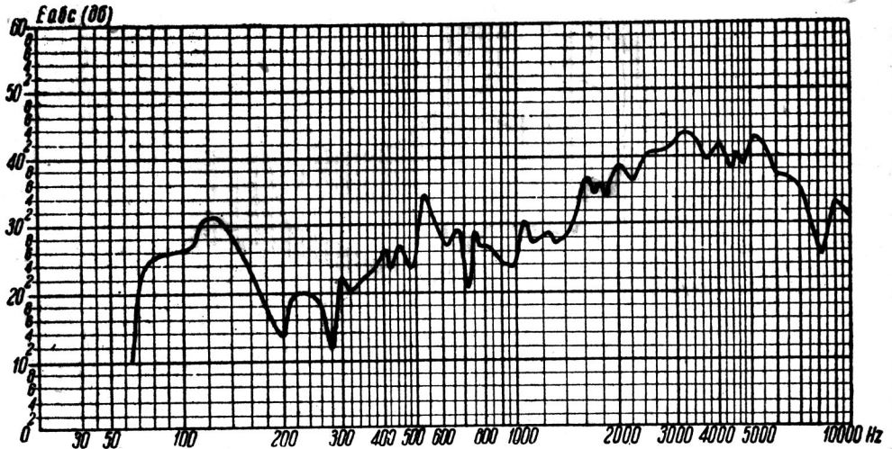
Рис. 24. Частотная характеристика абсолютной чувствительности громкоговорителя ГРА-2М (0 децибел — E_{abc} при P=1 бар, U=1 вольт, Z=1 ом)
