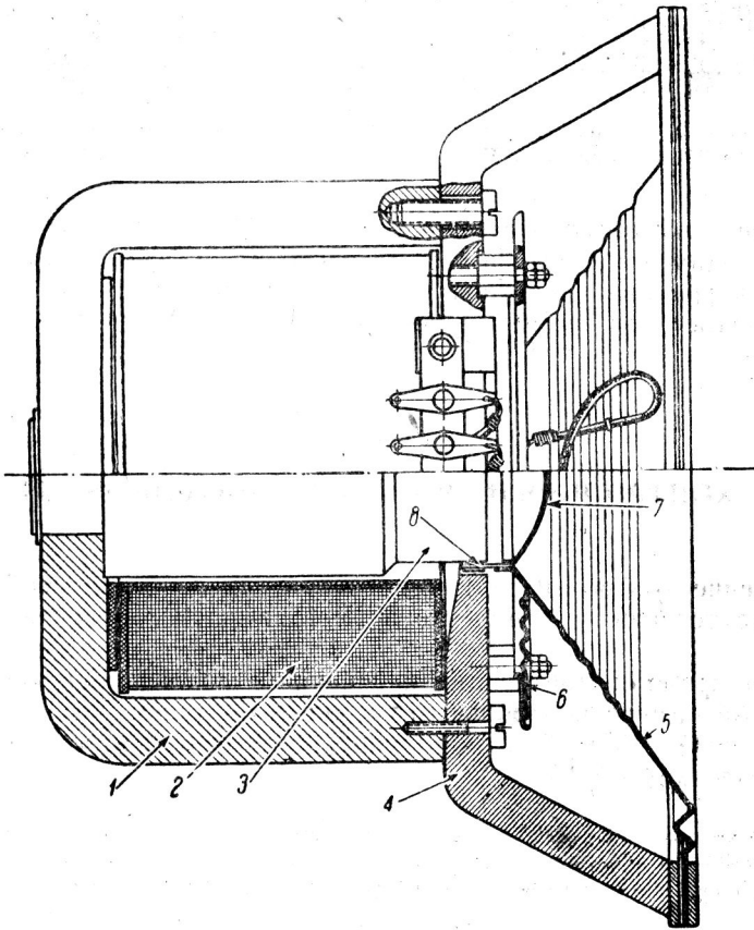
Рис. 23. Головка 1А-10 (эскизный чертеж конструкции)
