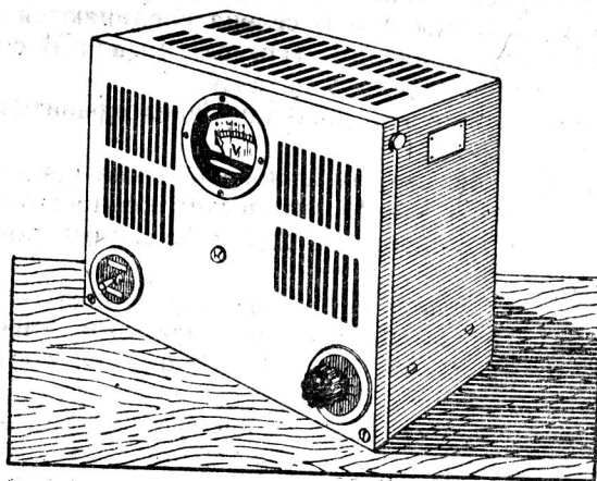
Рис. 17. Общий вид выпрямителя 1В-45
