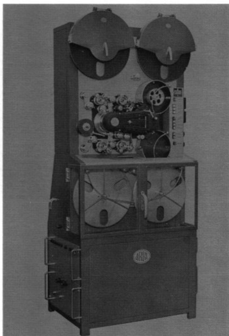
АРРИ кинокопировальный аппарат
