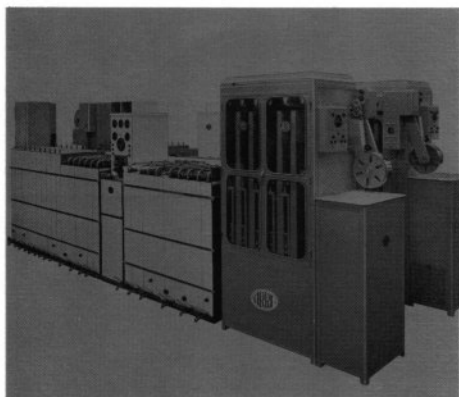
АРРИ проявочная машина
