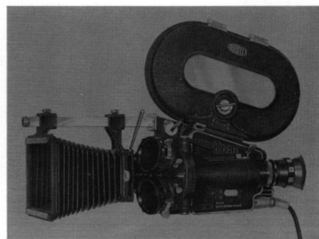
АРРИФЛЕКС 16 М
