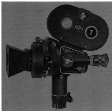
АРРИФЛЕКС 35 II С для 35-мм пленок
