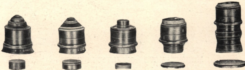
Комплект киносъемочных объективов в переходных оправках.
